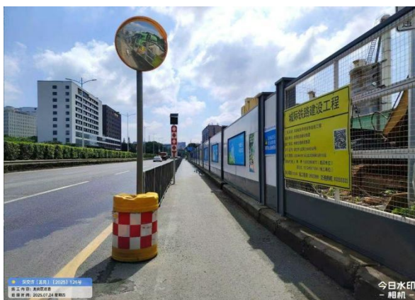
端头位置设置施工公示牌、防撞沙桶、凸面镜、通透式围挡等设施
